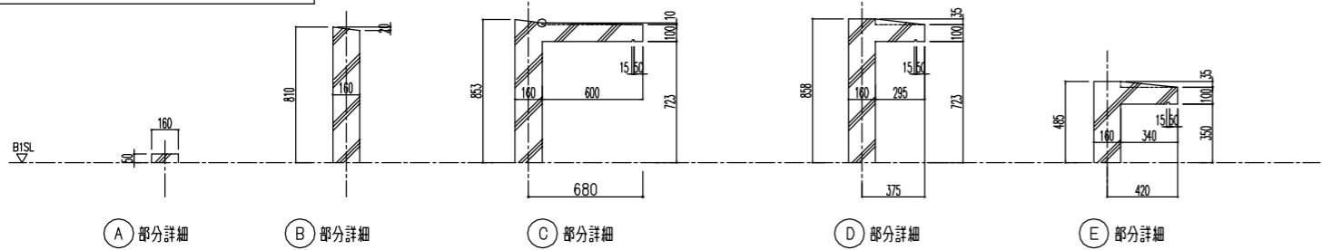
開口部立上り部分詳細図 1/20
